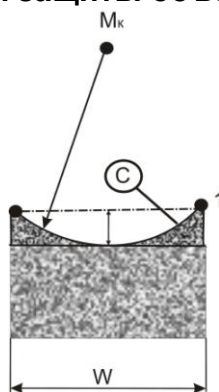
Рисунок 7.13 – Варианты защиты объектов на сложной кровле
