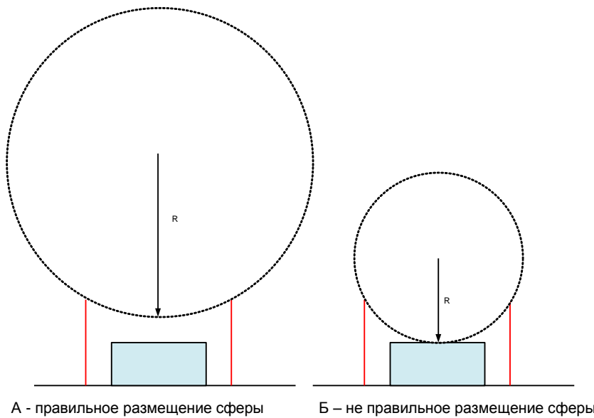
Рисунок 7.12 – Электрогеометрический метод качения сферы
