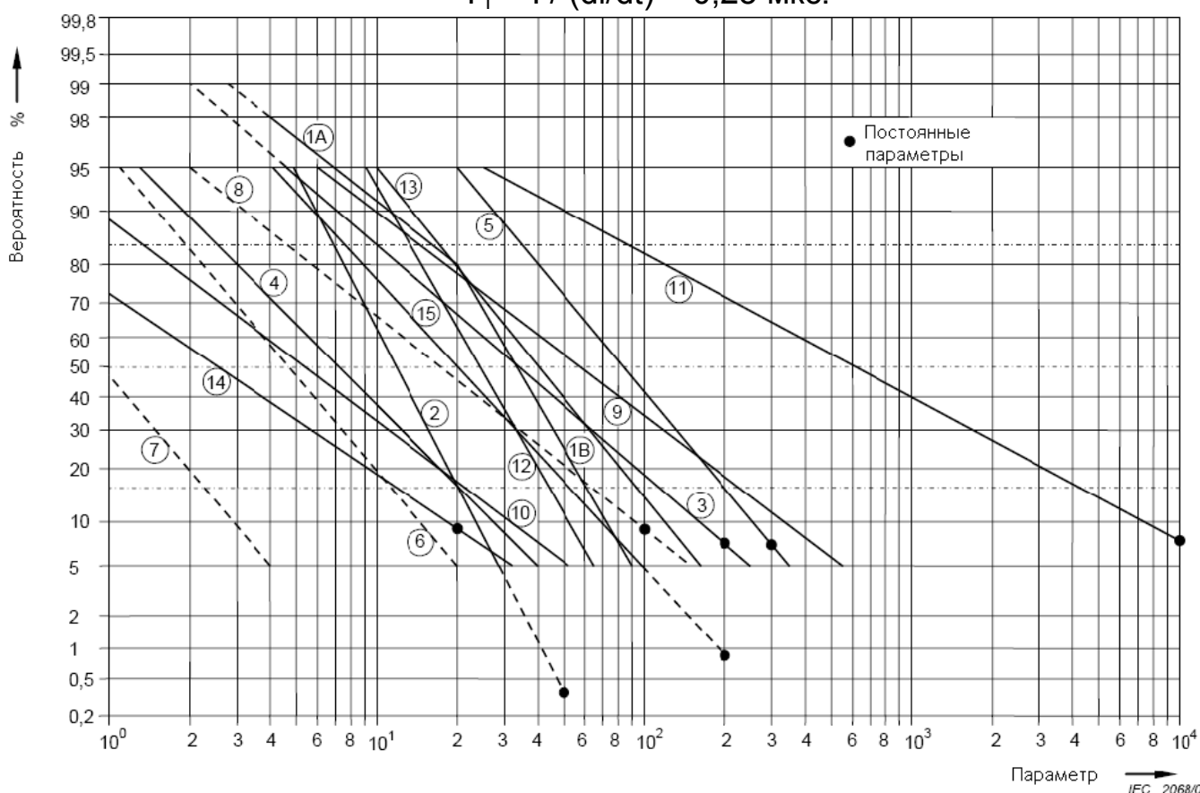
Рисунок 5.3 – Кумулятивное частотное распределение параметров тока молнии (прямые, проходящие через точки значений 95 % и 5 %)
