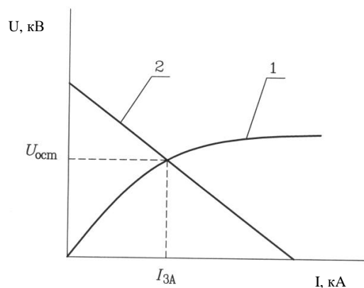
Рисунок 10.10 – Графическое определение тока через защитный аппарат
