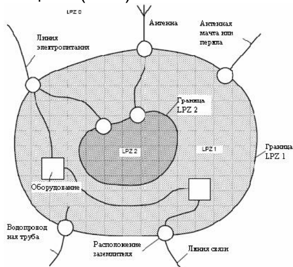
Рисунок 8.1 – Общий принцип деления на разные ЗМЗ: заземление входящих устройств напрямую или с помощью соответствующего ОПН
