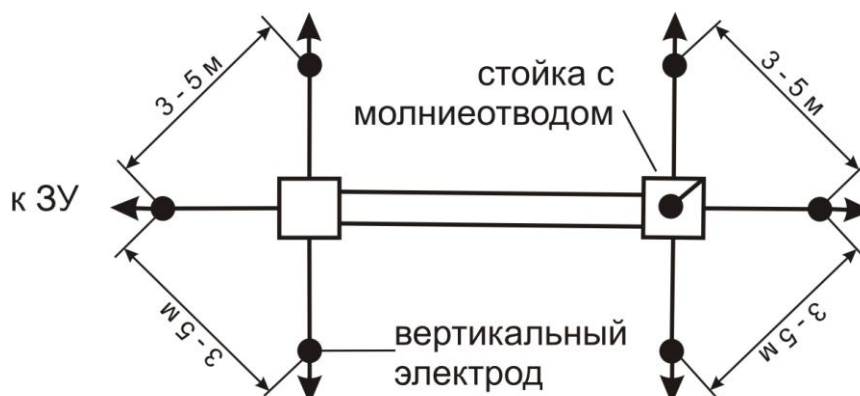
Рисунок 10.17 – Схема заземления молниеотвода, установленного на портале
