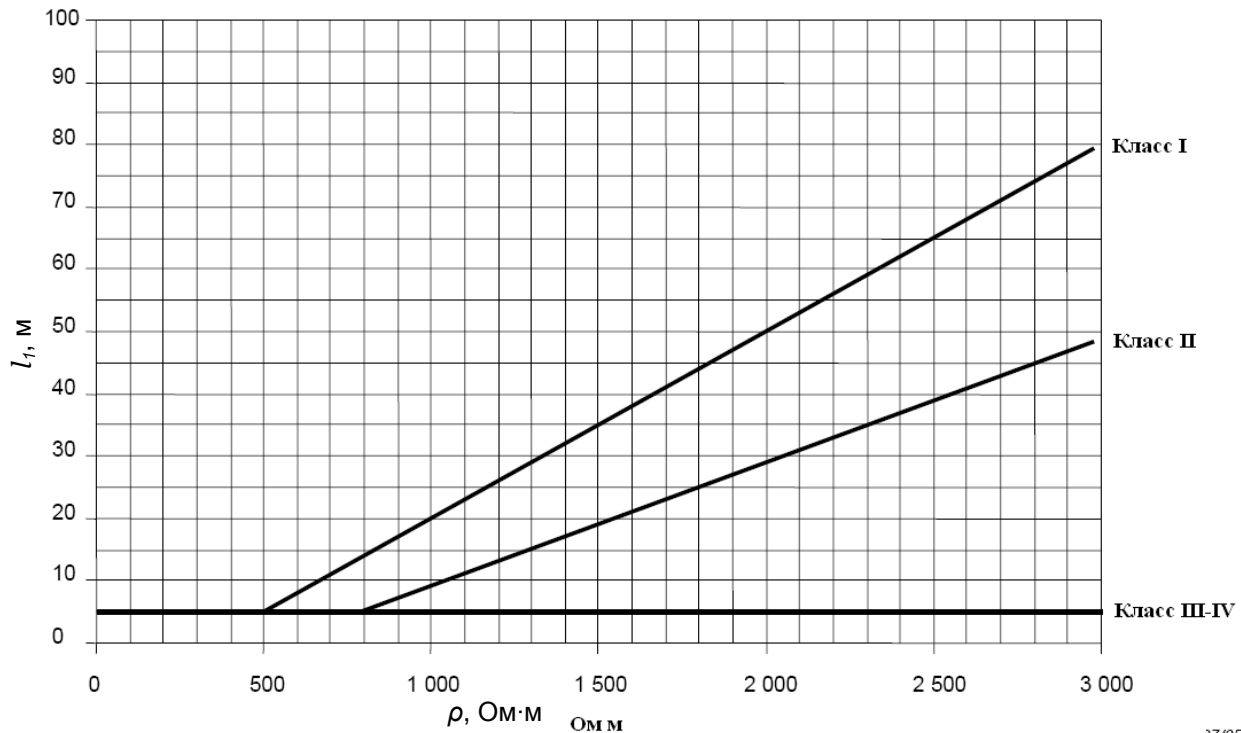
Рисунок 7.16 – Минимальная длина l_1 каждого заземляющего электрода в соответствии с классом СМЗ
