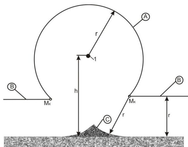
Рисунок 7.8 – Зона защиты тросового молниеотвода ( h > r )
