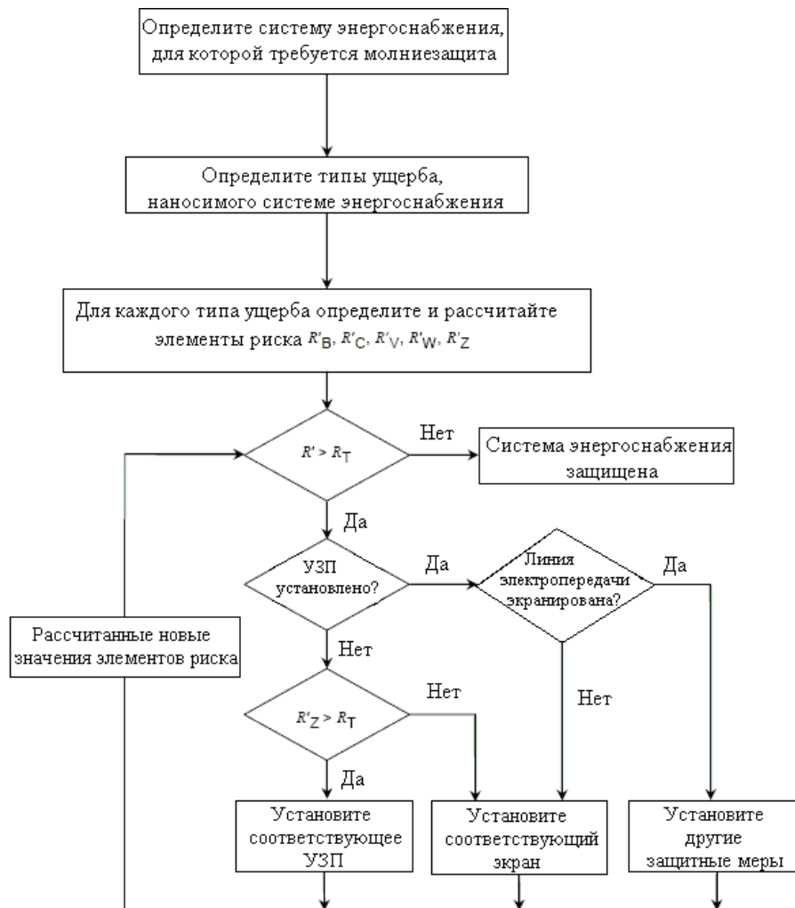
Рисунок 6.3 – Процедура выбора мер молниезащиты в системах энергоснабжения
