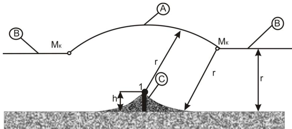
Рисунок 7.6 – Зона защиты тросового молниеприемника ( h \leq r )
