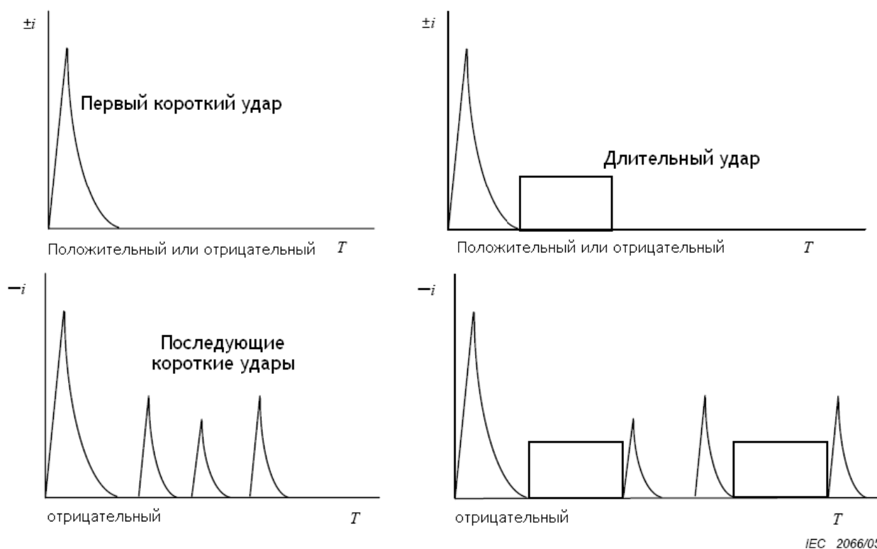
Рисунок 5.1 – Возможные компоненты нисходящих молний (типичных на равнинной местности и для невысоких зданий)
