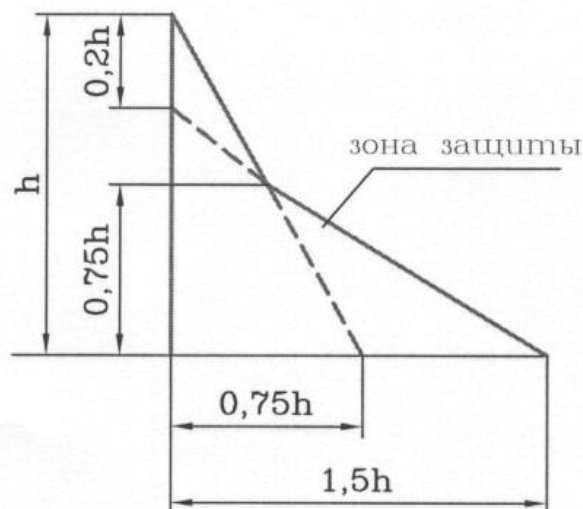
Рисунок 10.2 – Построение зоны защиты стержневого молниеотвода упрощенным методом
