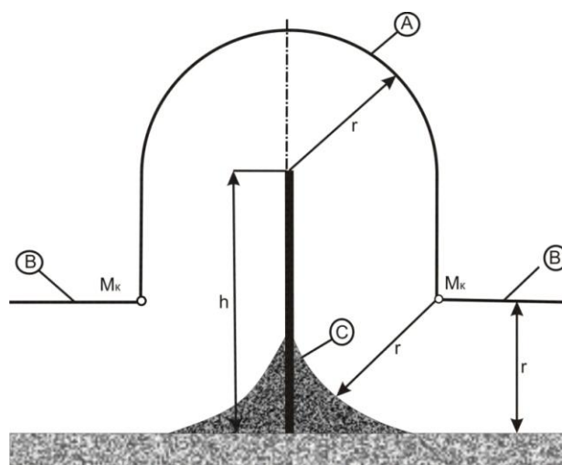
Рисунок 7.7 – Зона защиты башенного молниеотвода ( h > r )
