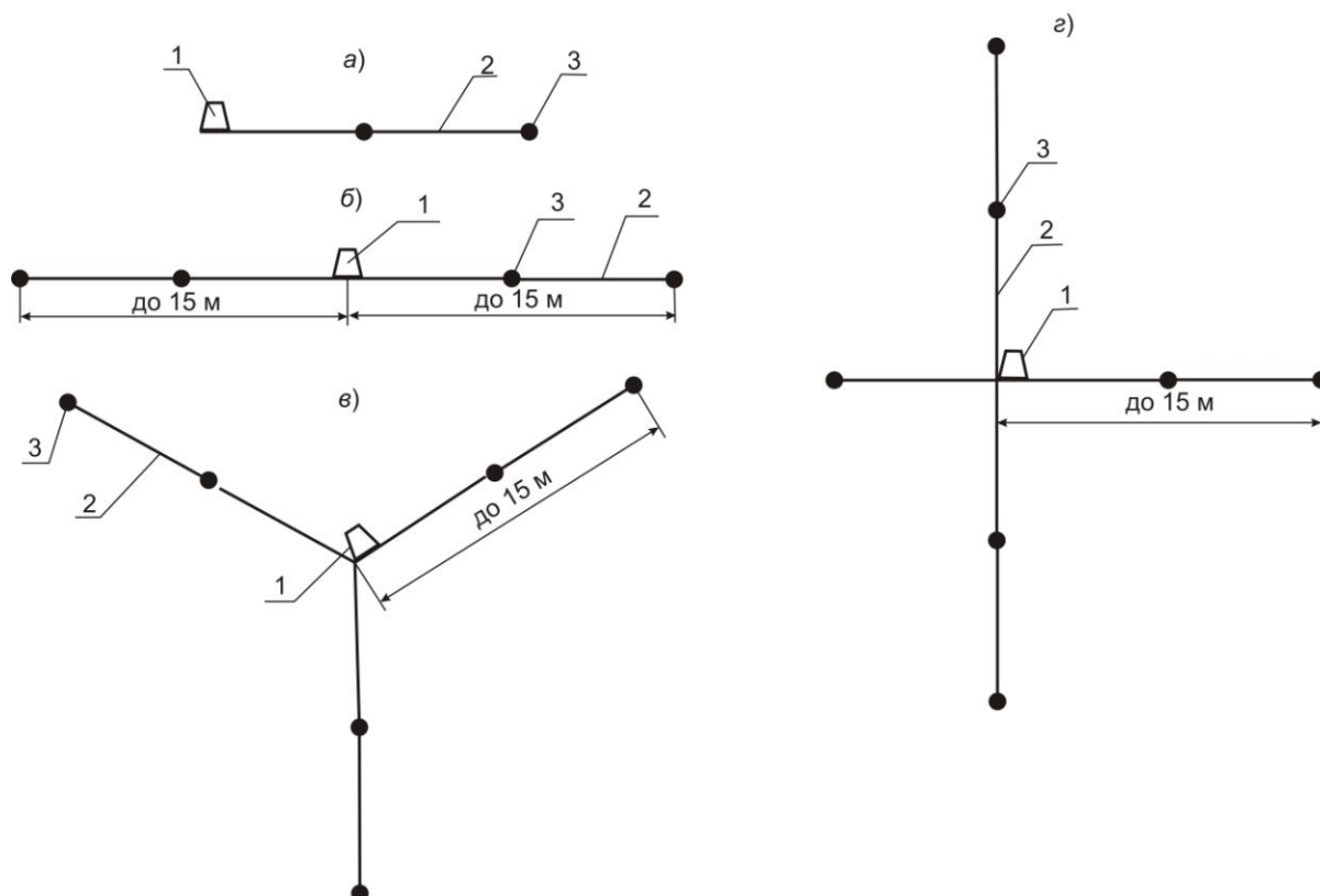
Рисунок 10.25 – Заземляющее устройство мачтовой трансформаторной подстанции 10/0,4 кВ
