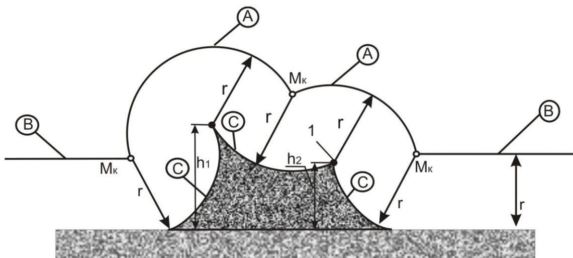
Рисунок 7.9 – Зона защиты двух тросовых молниеприемников ( h_2 < h_1 < r )
