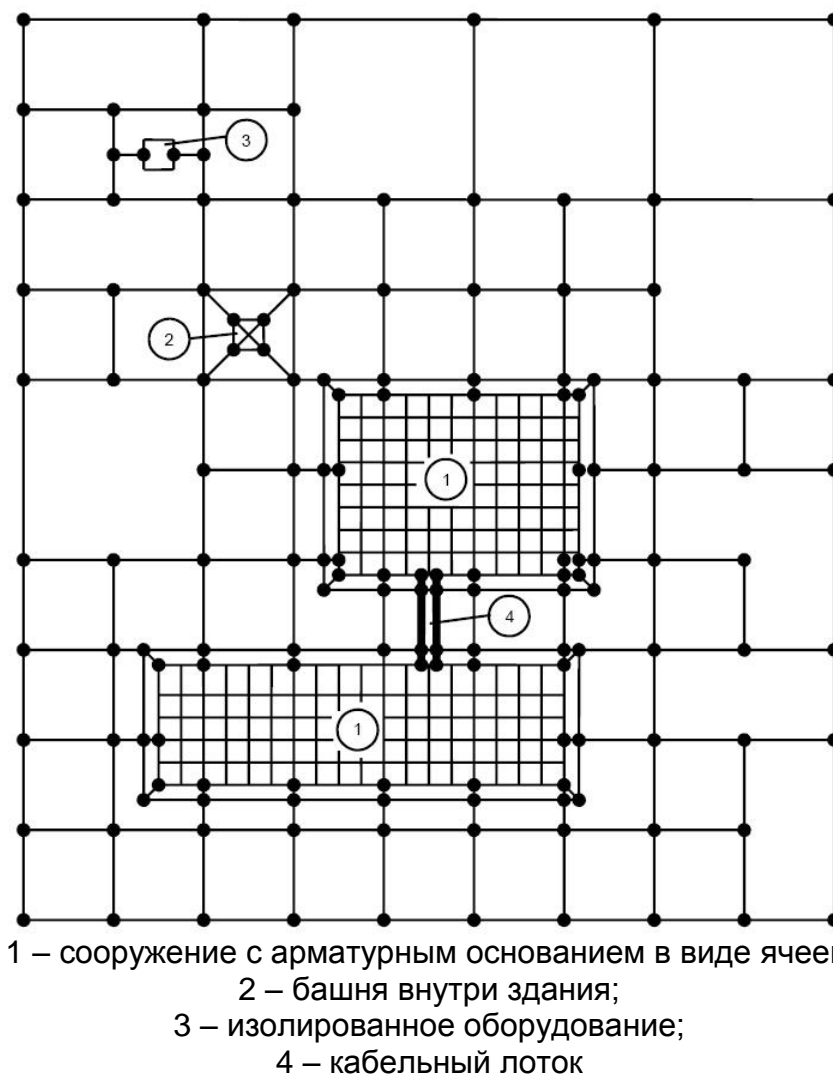
Рисунок 8.6 – Сетчатое заземляющее устройство здания или сооружения
