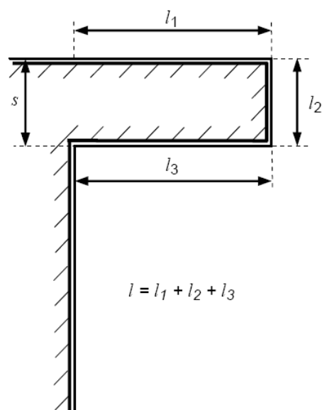
Рисунок 7.15 – Петля в токоотводе
