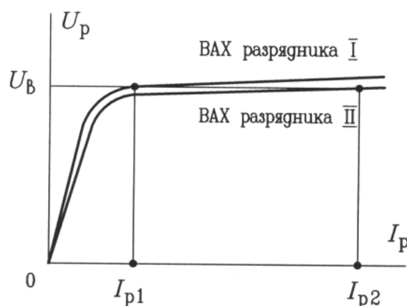
Рисунок 10.14 – Неравномерное распределение тока в параллельно включенных разрядниках
