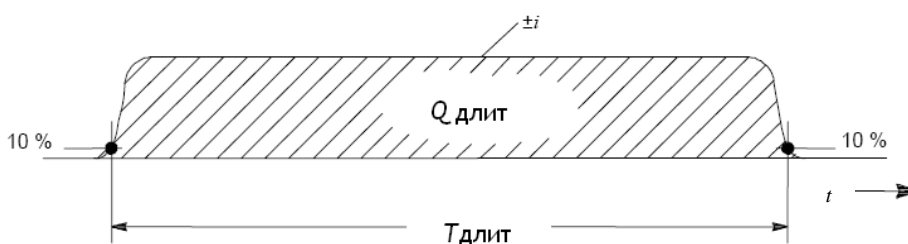
T_{\text{длит}} – длительность удара; Q_{\text{длит}} – заряд длительного удара (обычно 2 мс < T_{\text{длит}} < 1 с)
