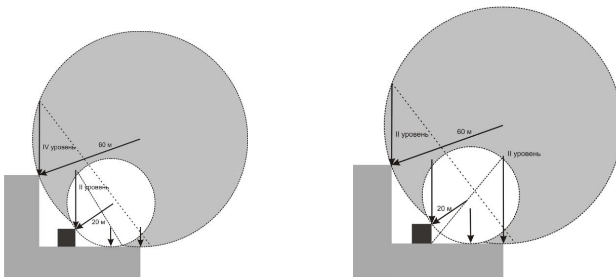
Рисунок 7.13 – Варианты защиты объектов на сложной кровле
