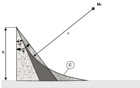
Рисунок 7.3 – Определение углов защиты
