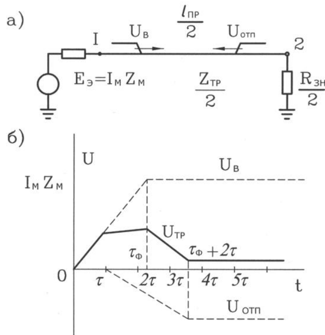
(а) – упрощенная эквивалентная схема
