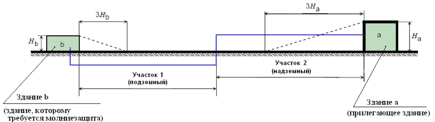
Рисунок 6.4 – Здания на концах линии
