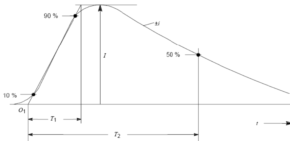
O_1 – виртуальный источник; I – пиковый ток; T_1 – время нарастания импульса; T_2 – время до половины значения (обычно T_2 < 2 мс)
