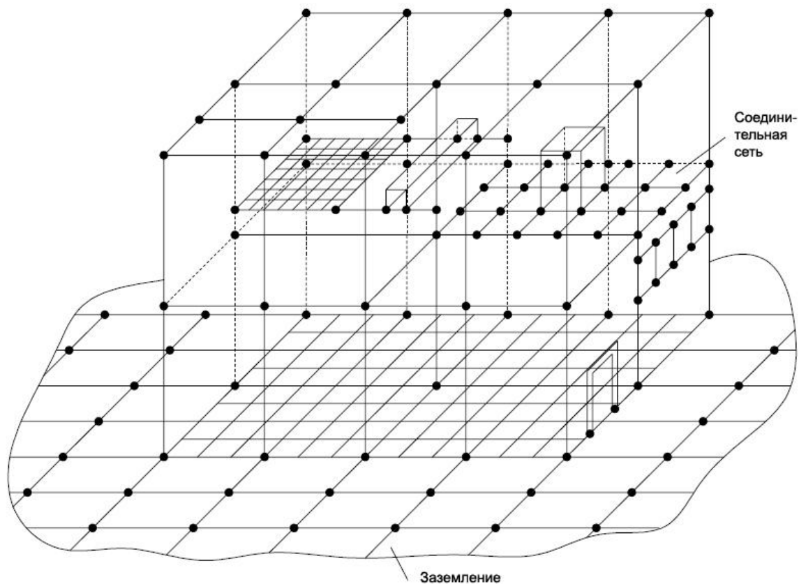
Рисунок 8.5 – Пример трехмерной системы заземления, заключающийся во взаимодействии соединительной сети и заземления
