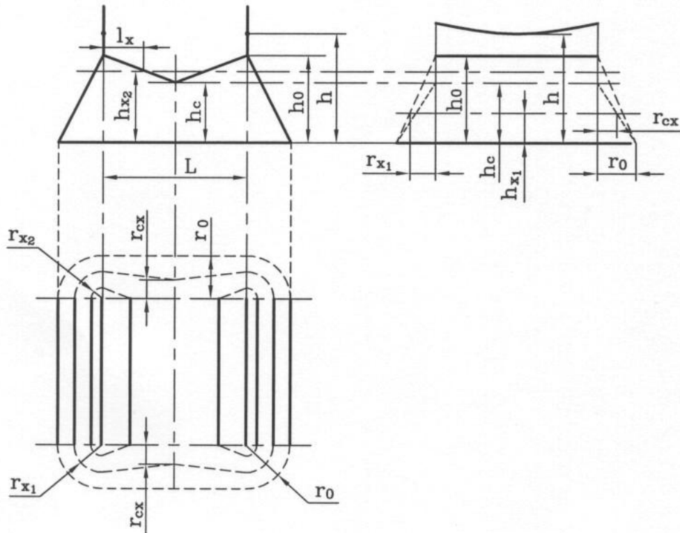
Рисунок 10.5 – Зона защиты двойного тросового молниеотвода
