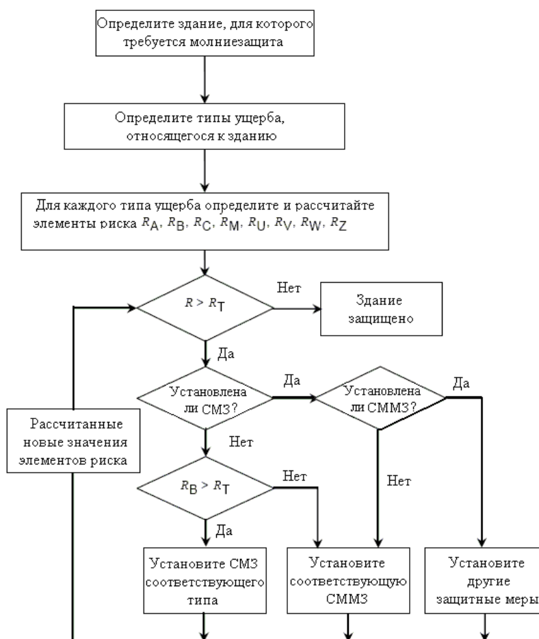
Рисунок 6.2 – Процедура выбора мер молниезащиты в зданиях
