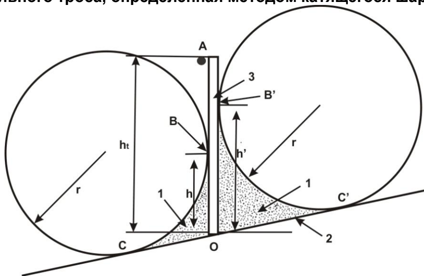
Рисунок 7.4 – Зона защиты молниеприемного стержня, мачты или горизонтального троса, определенная методом катящегося шара ( h_t < r )
