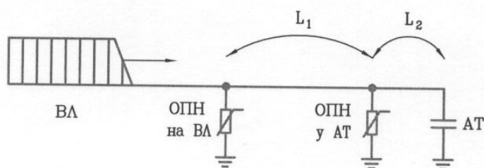
Рисунок 10.15 – Пример каскадной схемы защиты оборудования от перенапряжений
