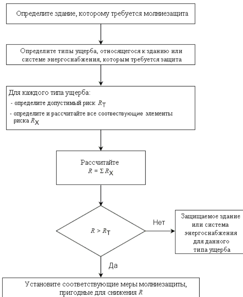
Рисунок 6.1 – Процедура принятия решения о необходимости молниезащиты
