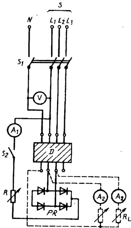
A_1 – амперметр действующих значений; A_2 – амперметр переменного тока; D – испытуемое УЗО – Д; PR – двухполупериодная мостовая схема на линейном напряжении; R – регулируемый резистор для дифференциального тока; R_L – активная нагрузка; S – источник переменного тока; S_1 – многополюсный выключатель; S_2 – однополюсный выключатель; V – вольтметр
